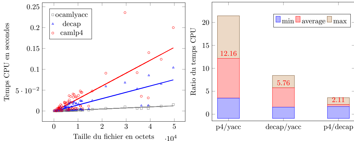
FIGURE 2 – Performances de la grammaire d'OCaml
